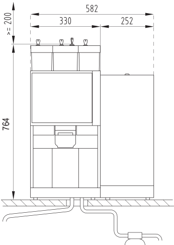
Frontansicht Maschine
