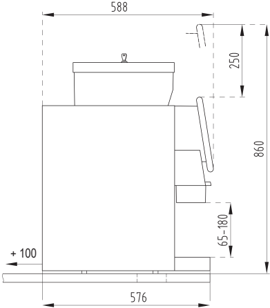
Seitenansicht Maschine
